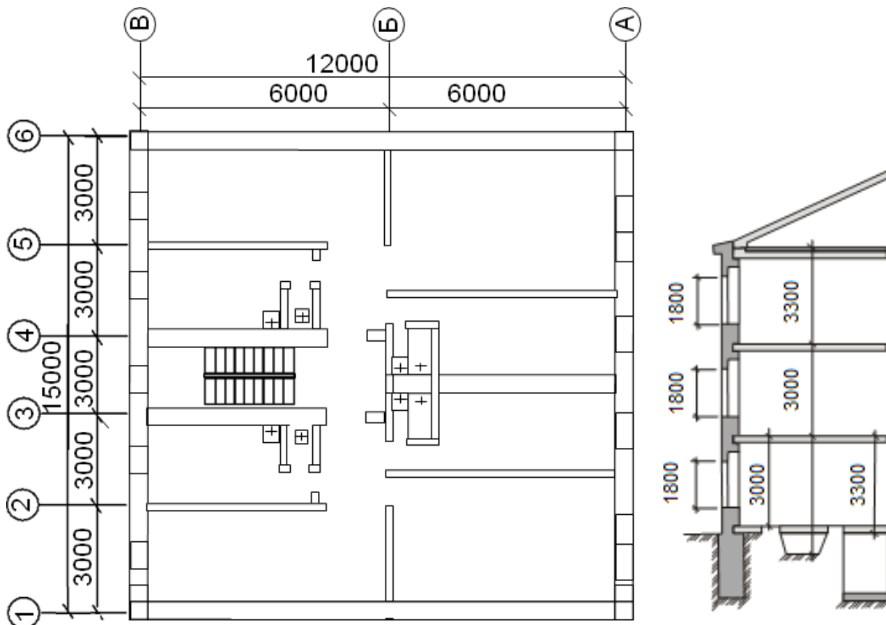
а) Рис. 1. План (а) и разрез (б) здания
